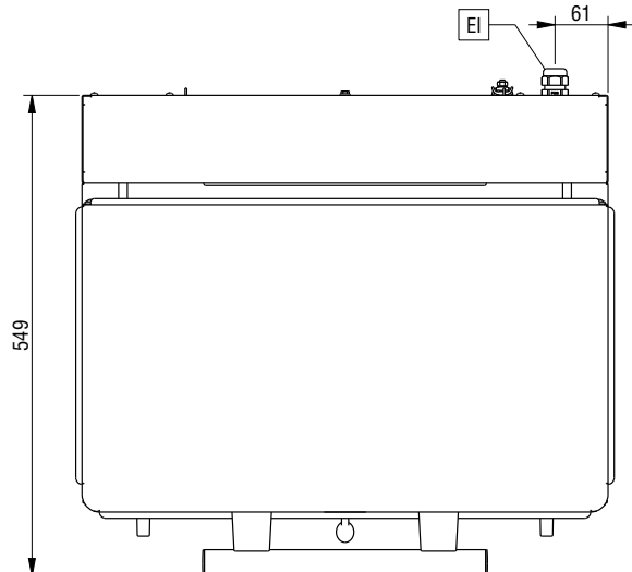
Päältä
